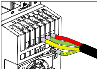
Рис. 4-8 Схема подключения кабеля двигателя
