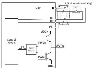
Рис. Е-2 Схема подключения функции STO
