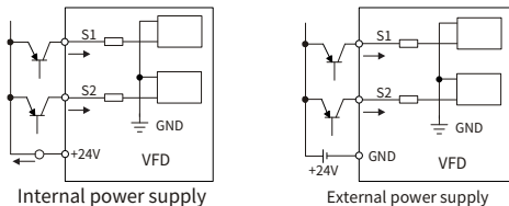
Рис. 4-13 Подключение PNP (источник)
