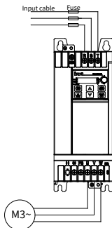
Рис. 4-17 Подключение плавких предохранителей
