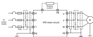
Рис. 4-6 Подключение главной цепи
