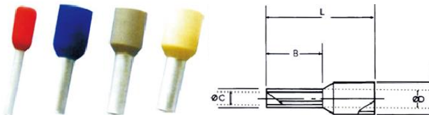
Рисунок D-1 Внешний вид и размеры трубчатого изолированного наконечника GTVE
