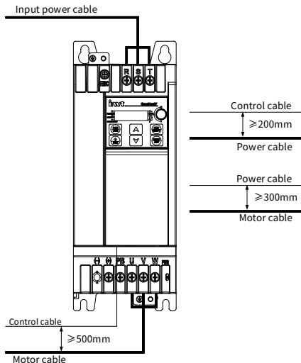
Рис. 4-5 Расстояния при прокладке кабелей
