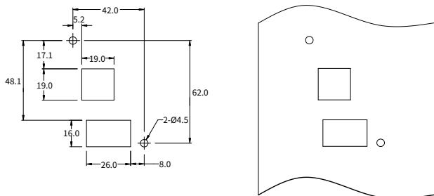
Рисунок D-5 Отверстия для крепления панели без кронштейна (ед. изм.: мм)
