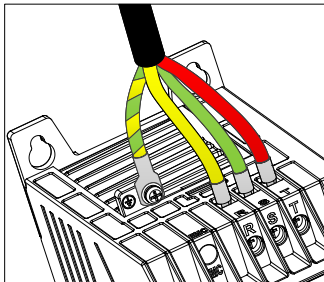
Рис. 4-7 Схема подключения входных силовых кабелей
