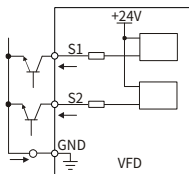
Рис 4-12 Подключение NPN (приемник)
