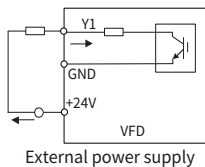
Рис. 4-14 Подключение клеммы Y1
