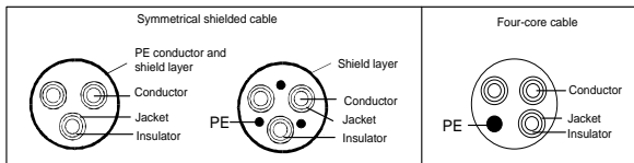
Рис. 4-4 Поперечное сечение кабеля
