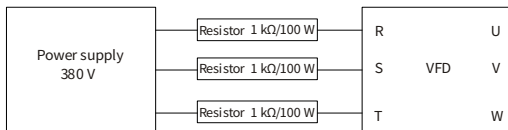
Рис. 9-1 Пример схемы зарядки ПЧ 380 В
