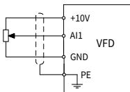
Рис. 4-15 Подключение аналоговых входных клемм
