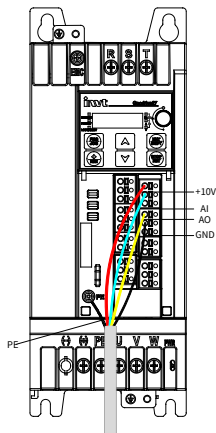
Рис. 4-16 Подключение экранирующего слоя PE
