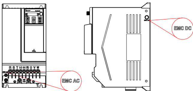
Рис. 4-2 Витн подключения EMC (D, E)
