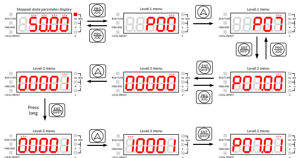
Рис. 5-4 Установка пароля
