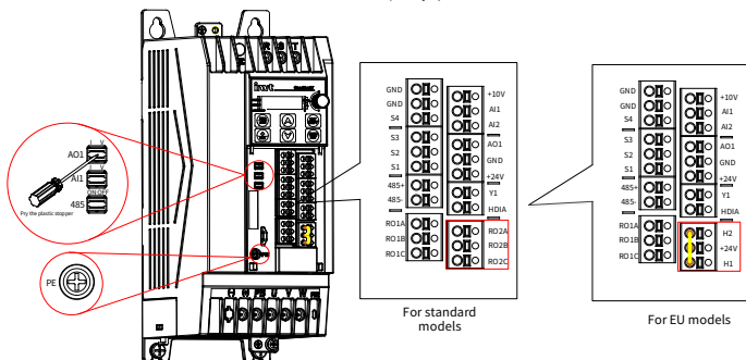
Рис. 4-11 Клеммы цепи управления
