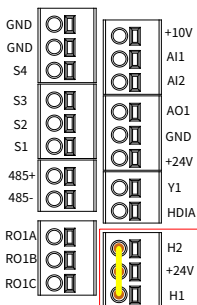
Рис. Е-2 Схема подключения функции STO
