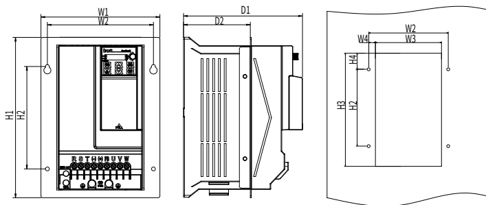
Рисунок С-6 Размеры и положение отверстий конструкции D
